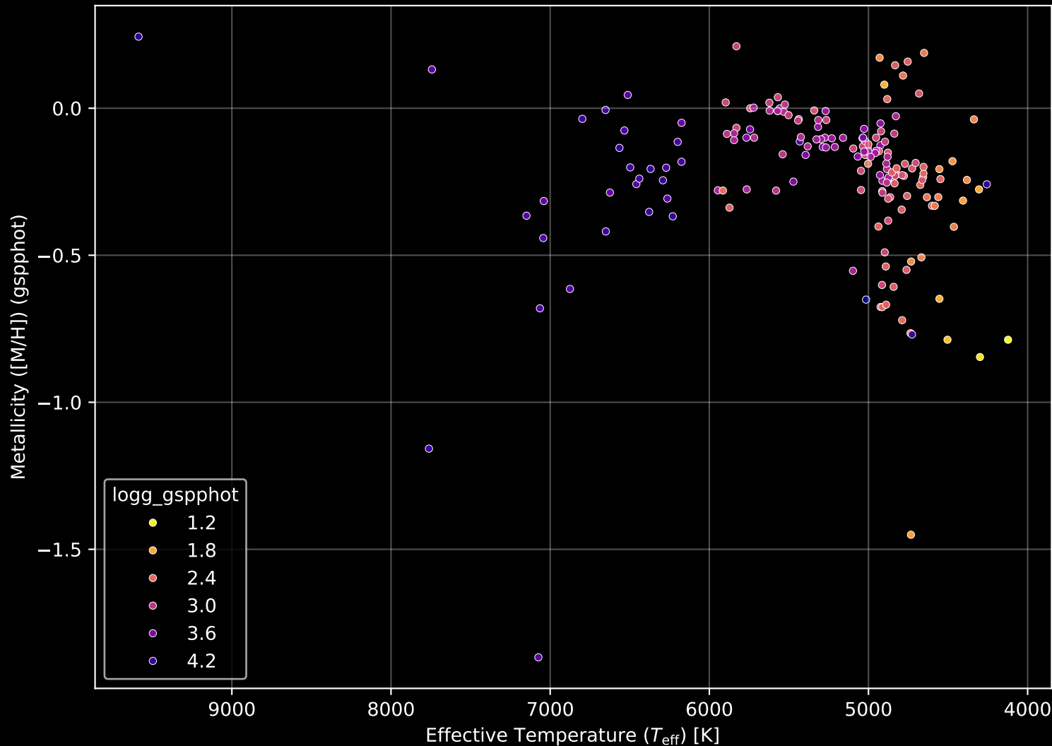
APOGEE DR17 Field: [075+35] Stellar Population Parameters (n= 176)
